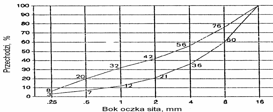
Rysunek 1. Krzywe graniczne uziarnienia kruszywa do betonu
