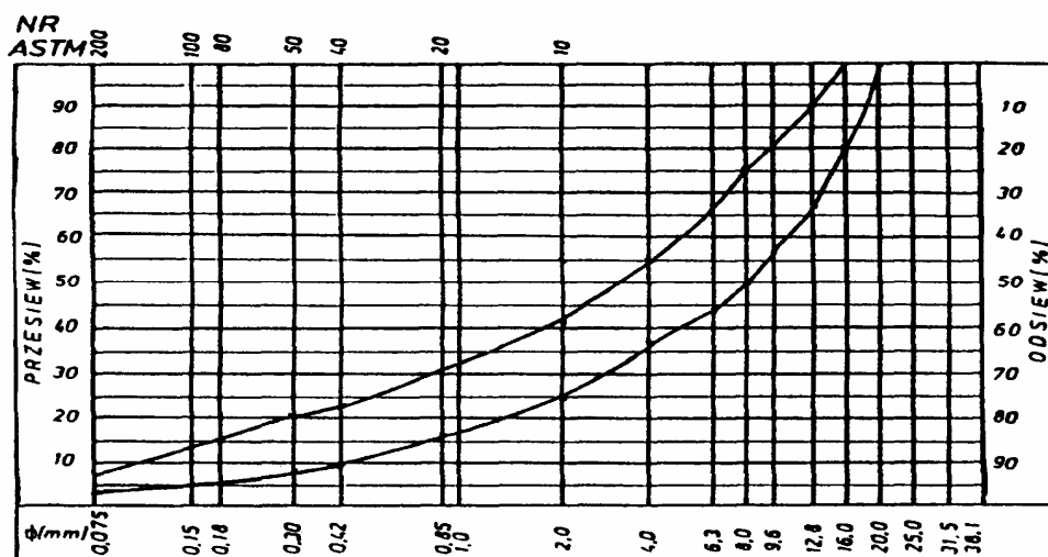
Rys. 3. Krzywe graniczne uziarnienia mieszanki mineralnej 0+16 mm do warstwy wiążącej z betonu asfaltowego dla KR 1-2
