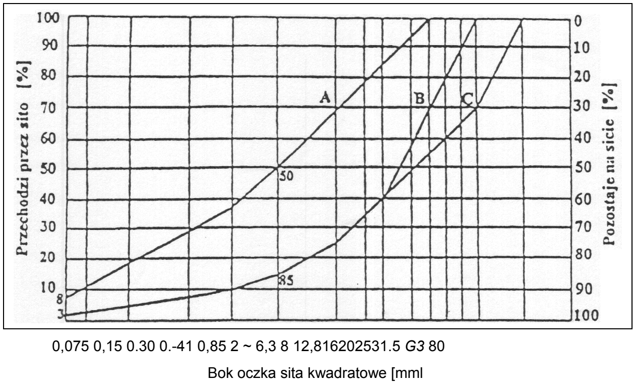
Rys. 1. Graniczne uziarnienie mieszanki mineralno-cementowo-emulsyjnej do podbudowy dróg o kategorii ruchu od KR3 do KR6
