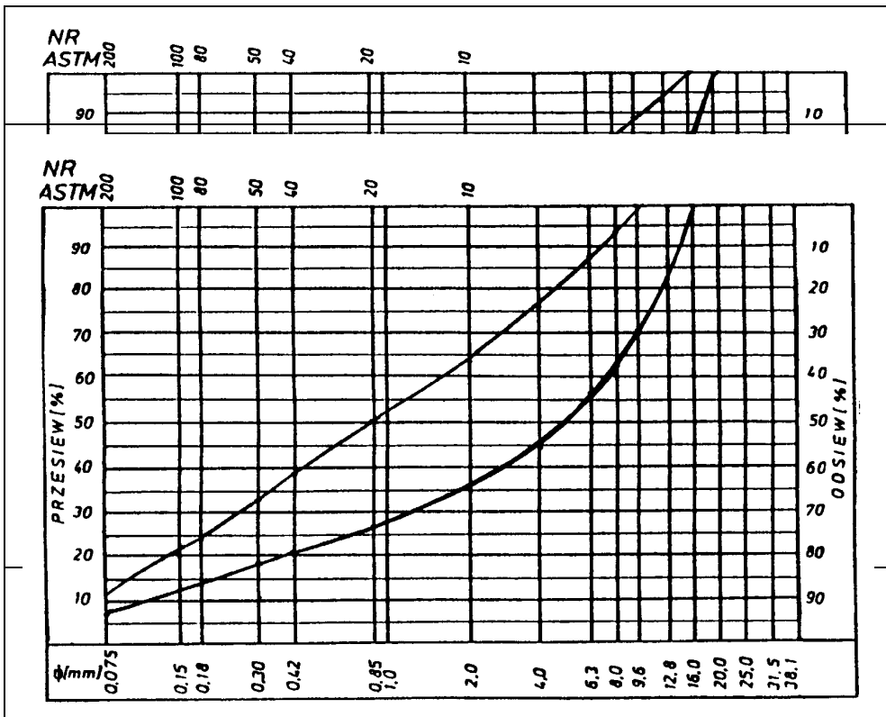
Rys. 2. Krzywe graniczne uziarnienia mieszanki mineralnej 0+16, 0+12,8 mm do warstwy ścieralnej z betonu asfaltowego dla KR 1-2
