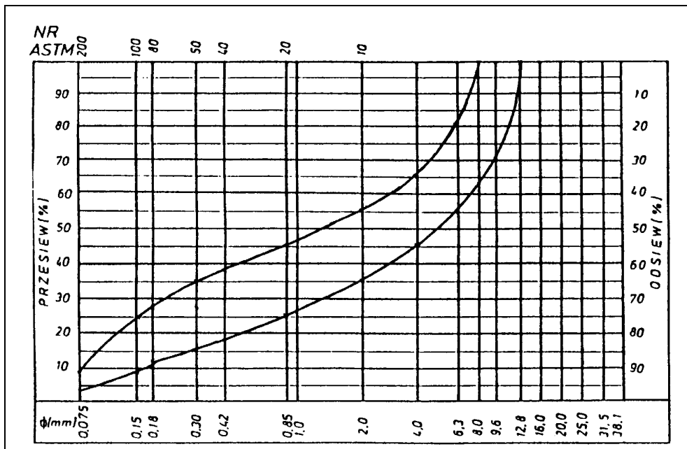
wyrównawczej i wzmacniającej z betonu asfaltowego dla KR 1-2 Rys. 10. Krzywe graniczne uziarnienia mieszanki mineralnej 0+12,8 mm do warstwy wiążącej, wyrównawczej i wzmacniającej z betonu asfaltowego dla KR 1-2
