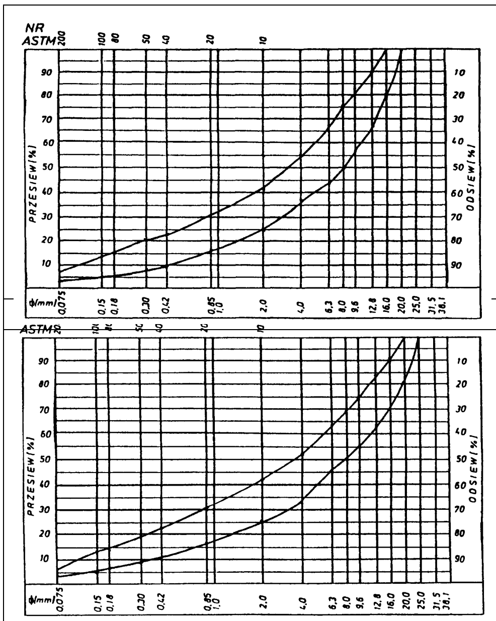
Rys. 11. Krzywe graniczne uziarnienia mieszanki mineralnej 0+25 mm do warstwy wiążącej,
