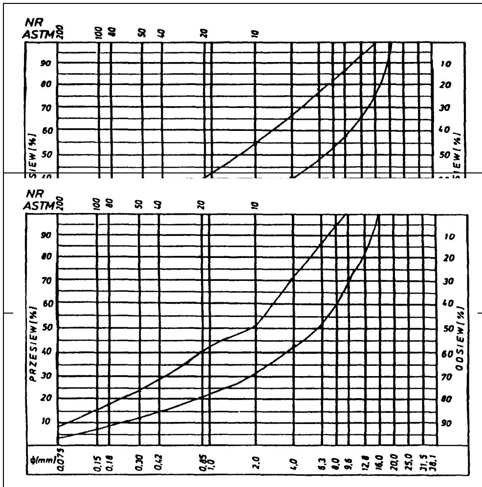
Rys. 9. Krzywe graniczne uziarnienia mieszanki mineralnej 0+16 mm do warstwy wiążącej,
