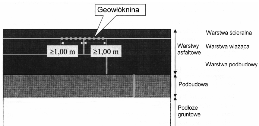
Rys. 6. Poszerzenie nawierzchni z wykonaniem stopni i wzmocnieniem geowłókniną
