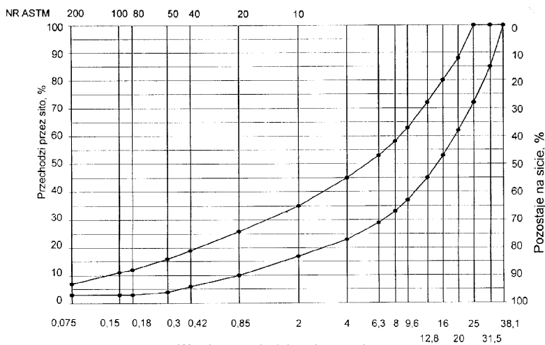
Krzywe graniczne uziarnienia mieszanki mineralnych do podbudowy z betonu asfaltowego przedstawiono na rysunkach od 1 do 7.
