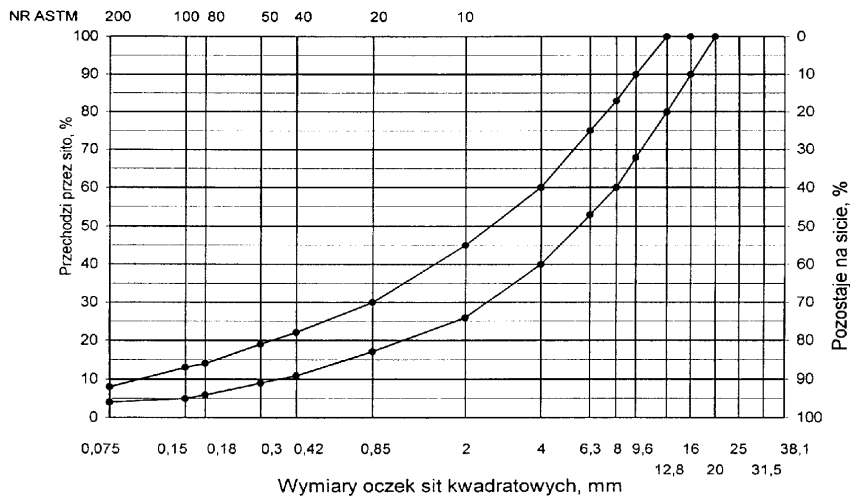
Rys. 3. Krzywe graniczne uziarnienia mieszanki mineralnej BA od 0 do 20 mm do podbudowy nawierzchni drogi o obciążeniu ruchem KR 1 lub KR 2
