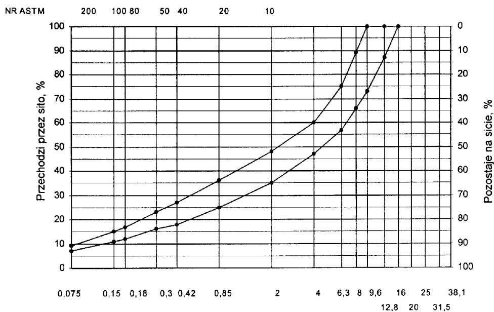
Rys. 4. Krzywe graniczne uziarnienia mieszanki mineralnej BA od 0 do 12,8 mm do warstwy ścieralnej nawierzchni drogi o obciążeniu ruchem od KR3 do KR6
