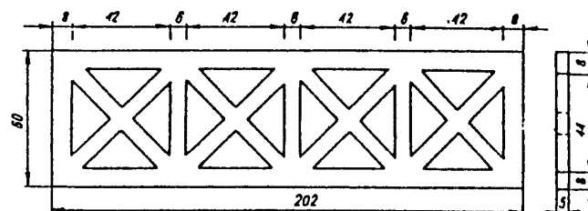
Deska ażurowa kombinowana 202 x 90 x 5 cm
