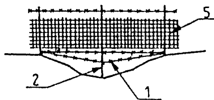
1 - dodatkowe druty kolczaste pod ogrodzeniem 2 - prześwit około 15 cm
